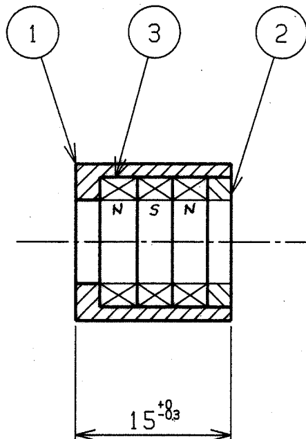
A-A断面
