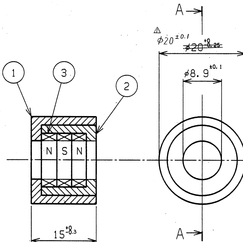
A-A断面
