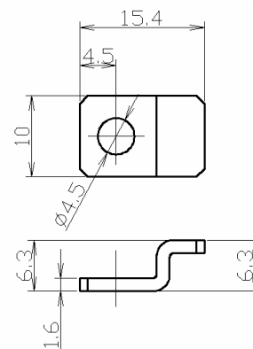
図2 取り付け金具
