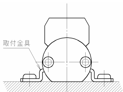
図3 取り付け断面
